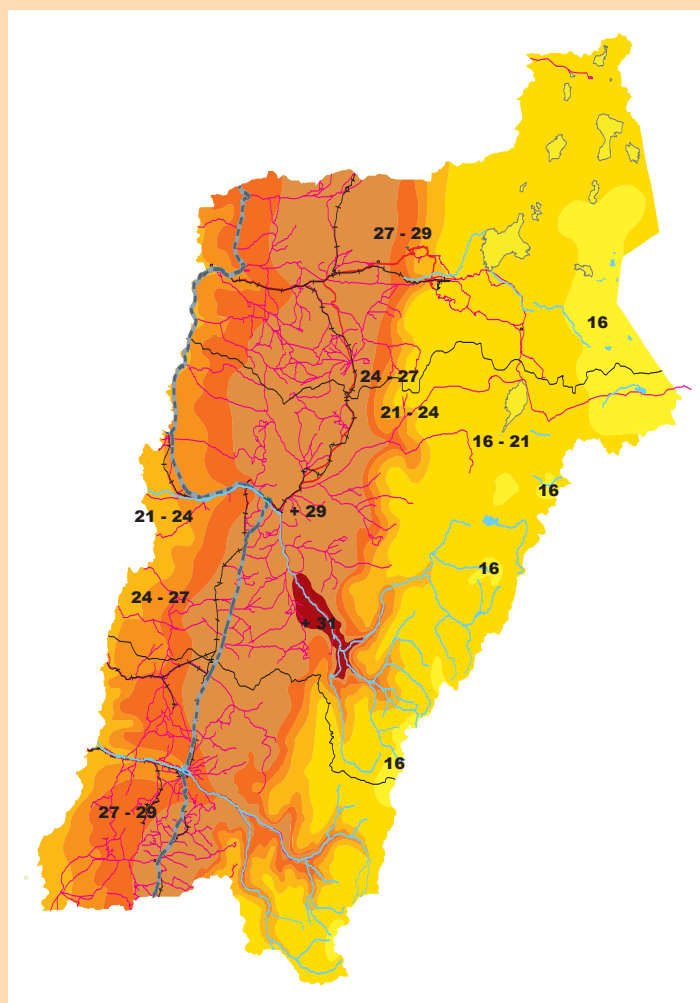
TEMPERATURA MÁXIMA MEDIA DE ENERO MEAN MAXIMUM TEMPERATURE OF JANUARY
